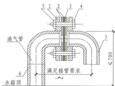
通气管安装剖面图
