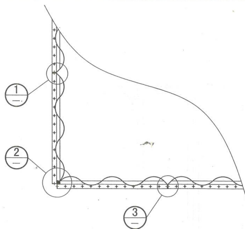
水箱模板连接示意图（俯视）
