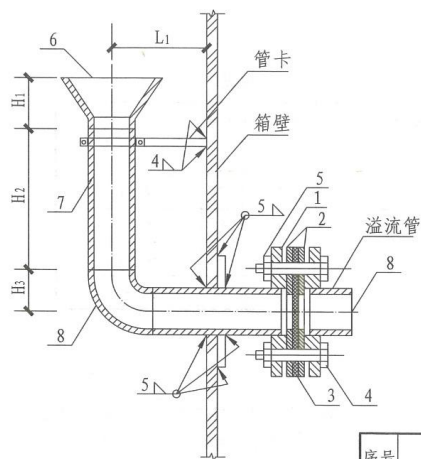
溢流管安装剖面图
