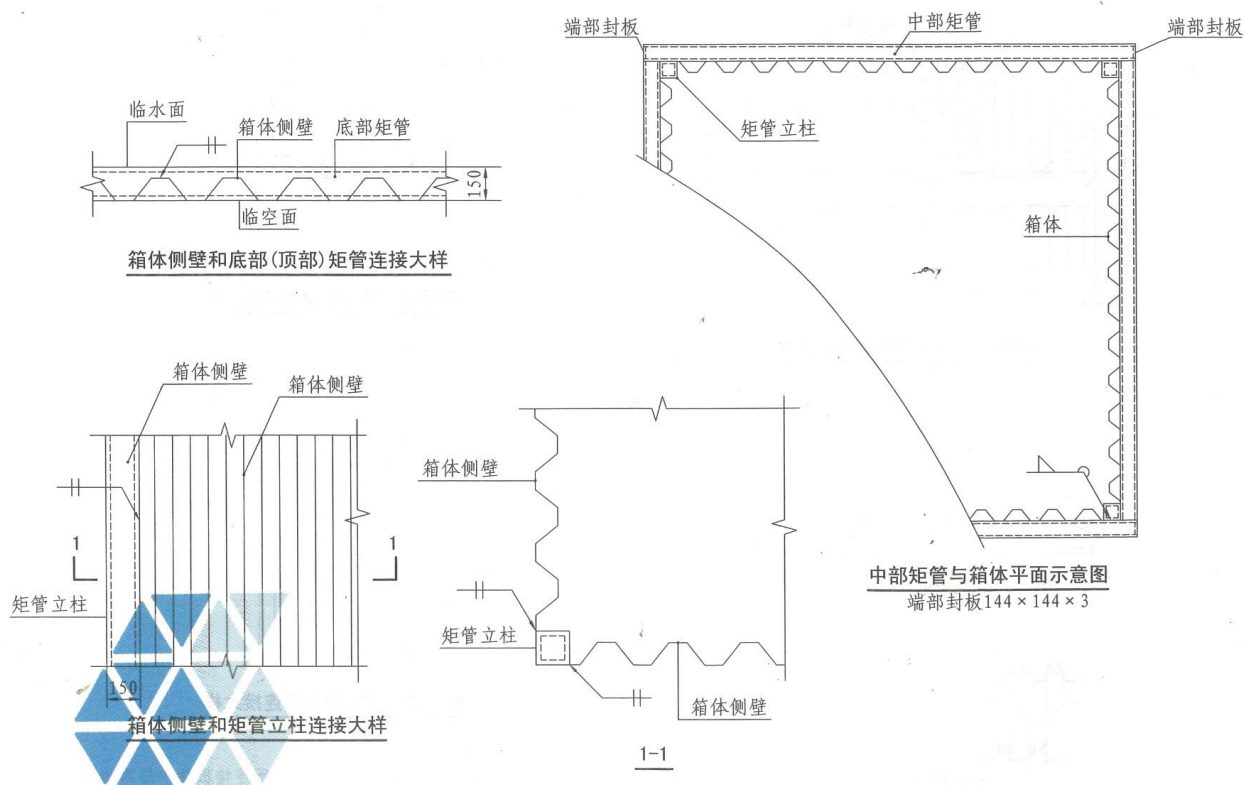
焊接式消防水箱箱体与矩管连接图 (一)
