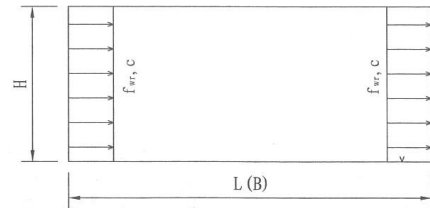
图9 水箱水平动水压力图
