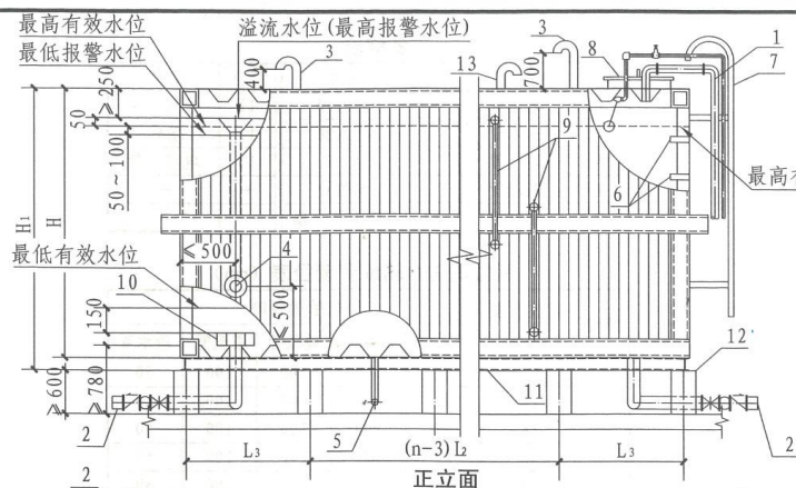
正立面图
