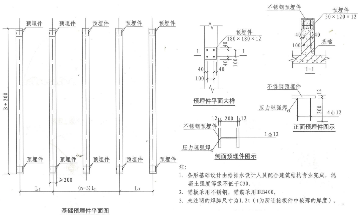
装配式弧肋板消防水箱基础图 (一)
