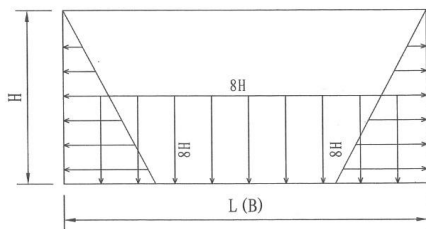
图10 水箱的竖向动水压力图
