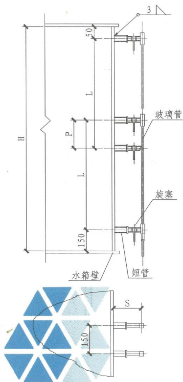
玻璃管液位计安装图
