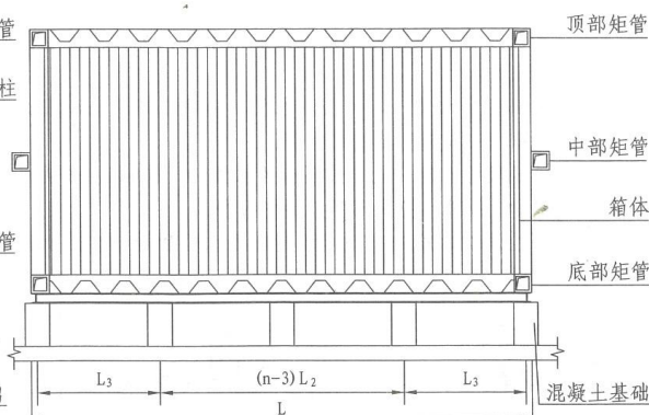
图5 水箱剖面图
