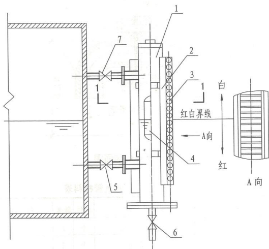
磁耦合液位计安装图
