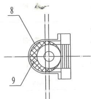
1-1剖面图 (保温式结构)
