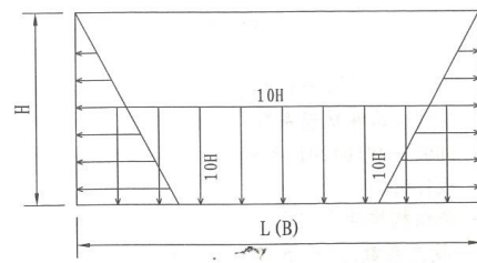
图8 水箱静水压力图
