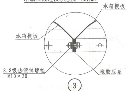
装配式弧肋板消防水箱连接图
