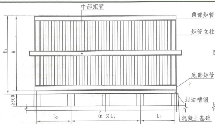
图3 水箱正立面图
