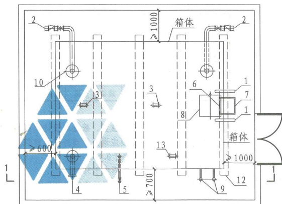
消防水箱水箱间平面布置图
