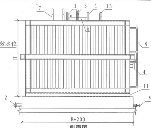
侧面图
