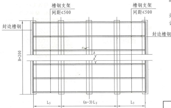
图4 水箱底部平面图
