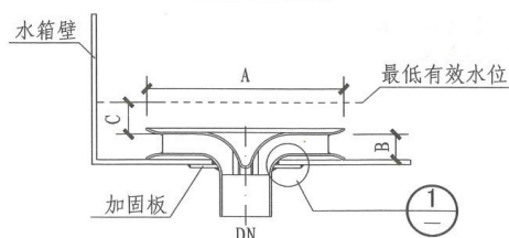
旋流防止器倒装图
