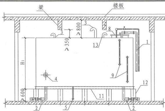
1-1剖面示意图
