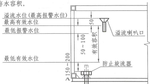
图1 水位示意图
