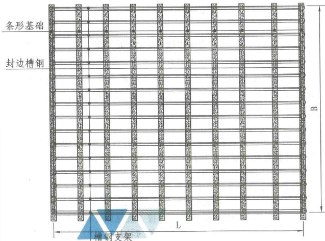
图7 约束示意图
