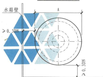
平面安装尺寸图
